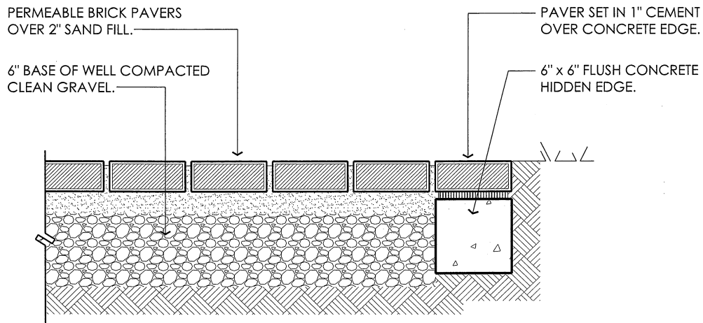
SECTION THRU PAVER EDGE - HIDDEN CURB
